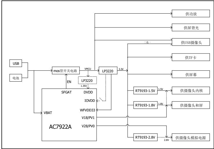
电源结构示意图
