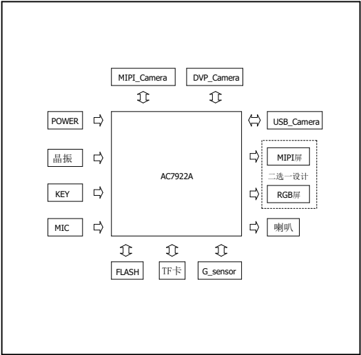
主控及外围功能模块
